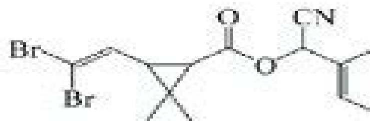
Deltamethrin
