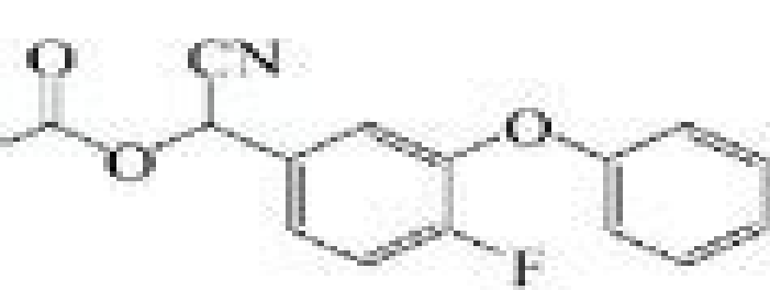
Cyfluthrin
