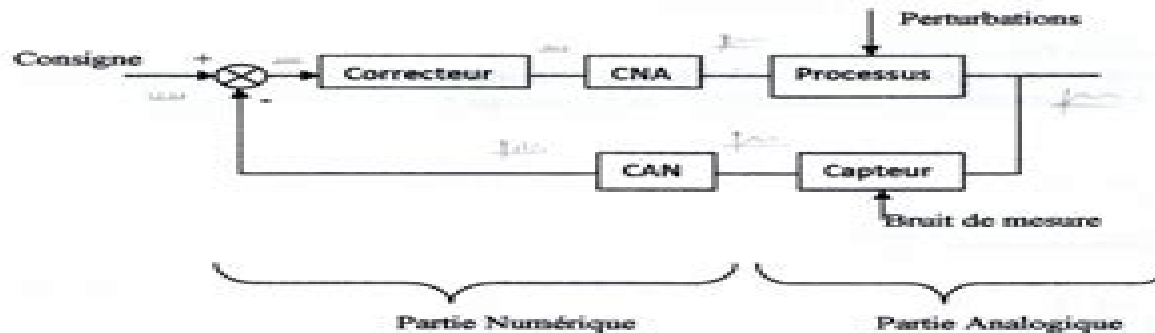
Fig. 1 Système à commande numérique.
