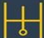
Uranus
