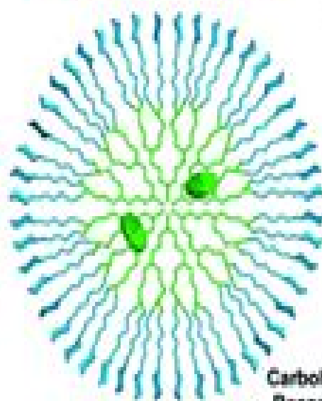
Glycodendrimers
