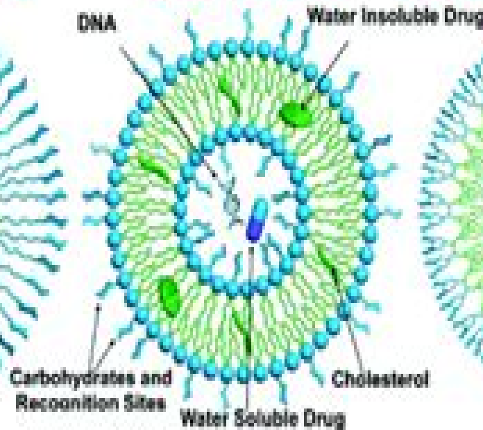
Glycoliposomes
