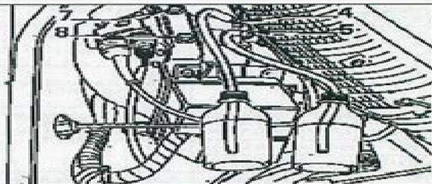
Purga del circuito de frenos. 4, 5, 7 y 8. Tornillos de purga del bloque hidráulico.
